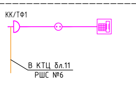
Структурная схема телефонной связи
