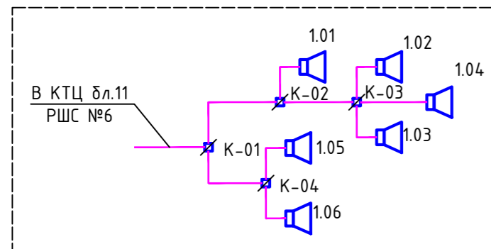
Командно-поисковая связь
