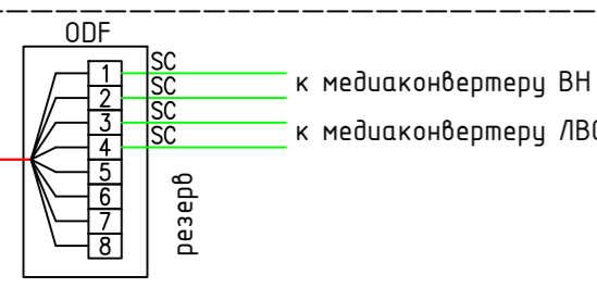
Схема разварки оптического кабеля в ТШ1
